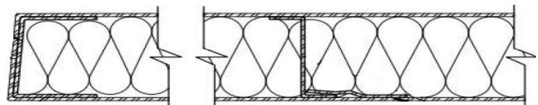
(Option soudure continue)
